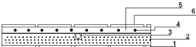
Joonis 2. Remonditavaale põrandale paigaldamine
